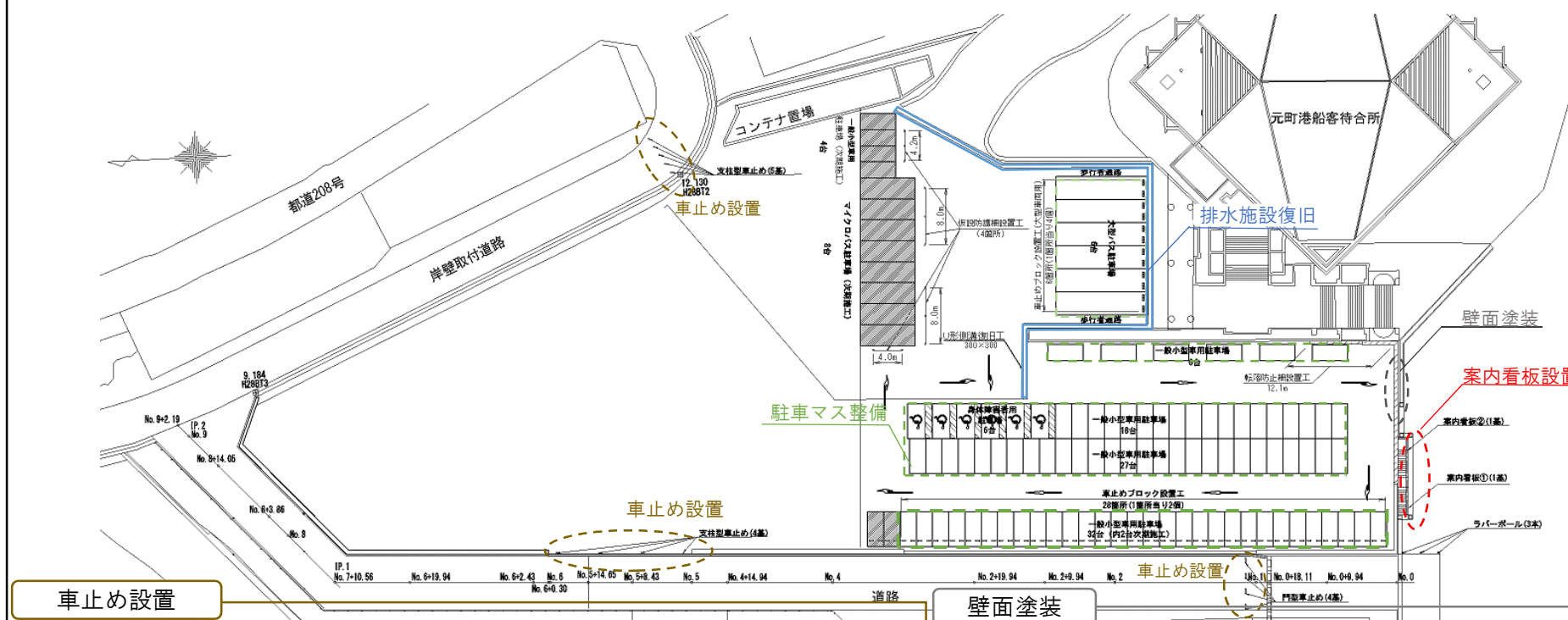
排水施設復旧
