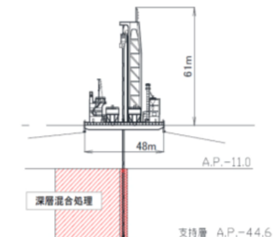
深層混合処理打設状況図
