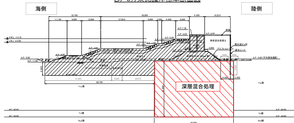
Dブロック東側護岸標準断面図
