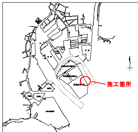
深層混合処理打設状況図
