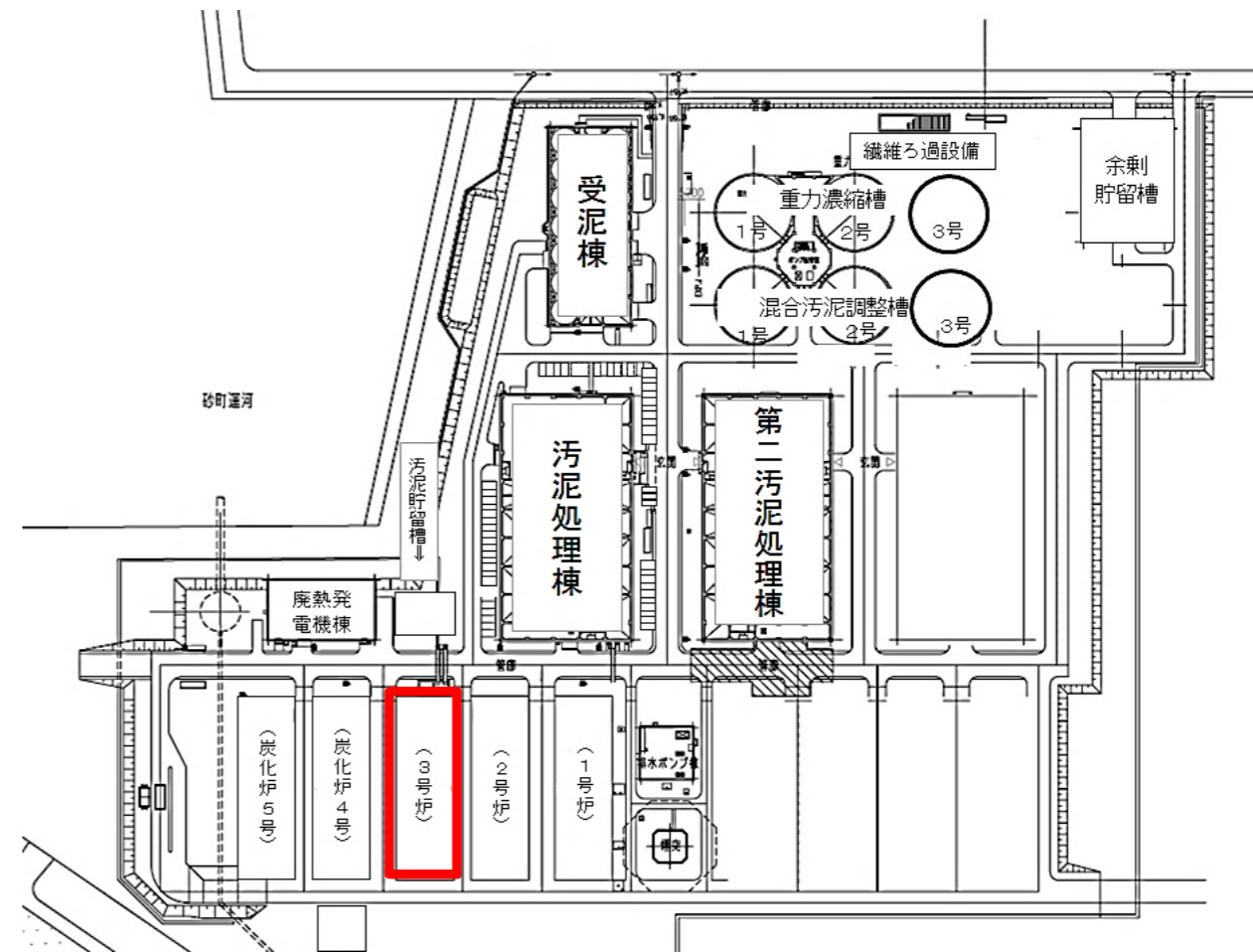
平面図(東部スラッジプラント) 施工箇所
