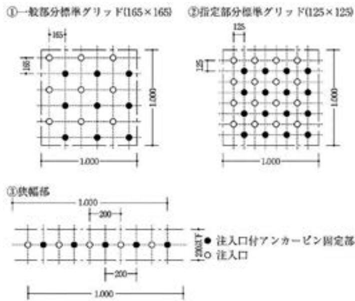
図24.4.4 標準グリッド(mm)
