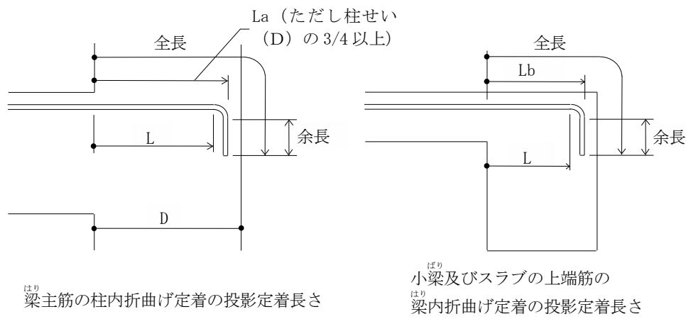
図 5.3.3 折曲げ定着の方法
