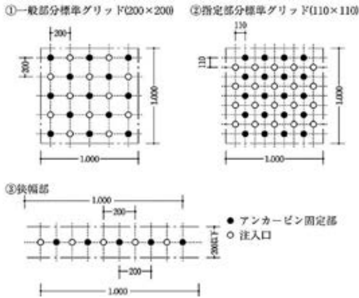
図24.4.2 標準配置グリッド(mm)
