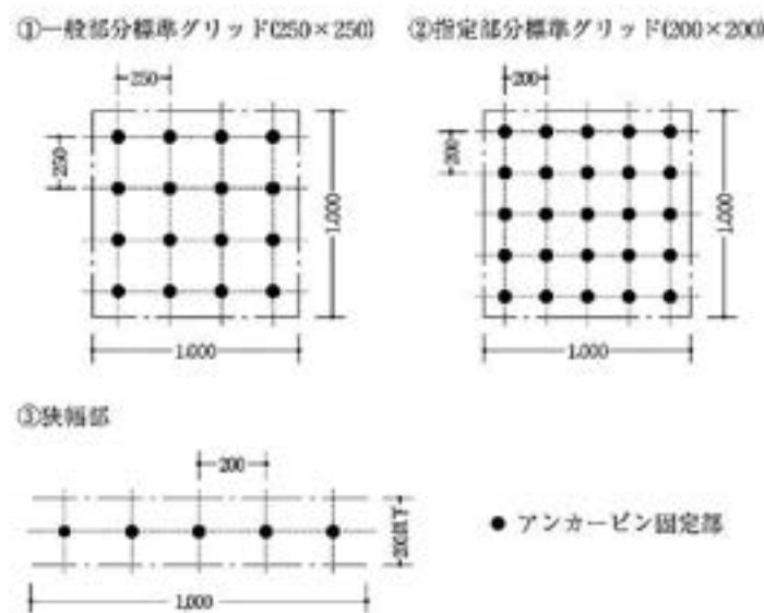
図24.4.1 標準配置グリッド(mm)
