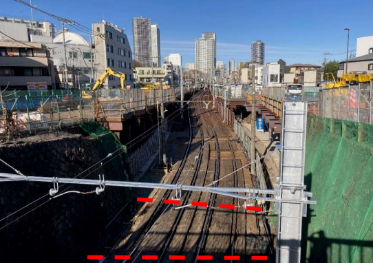
①施工箇所：発進立坑 (目白通り:千登世小橋北側)
