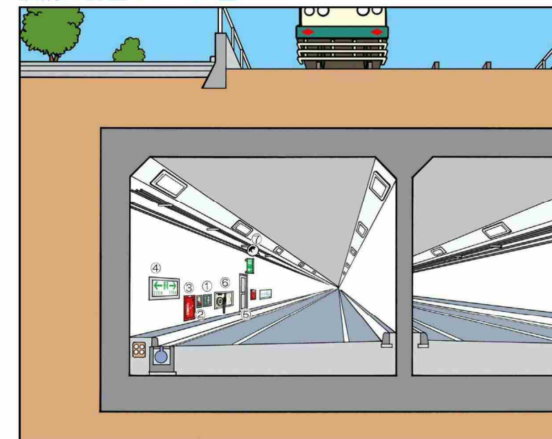
設備の配置イメージ図
