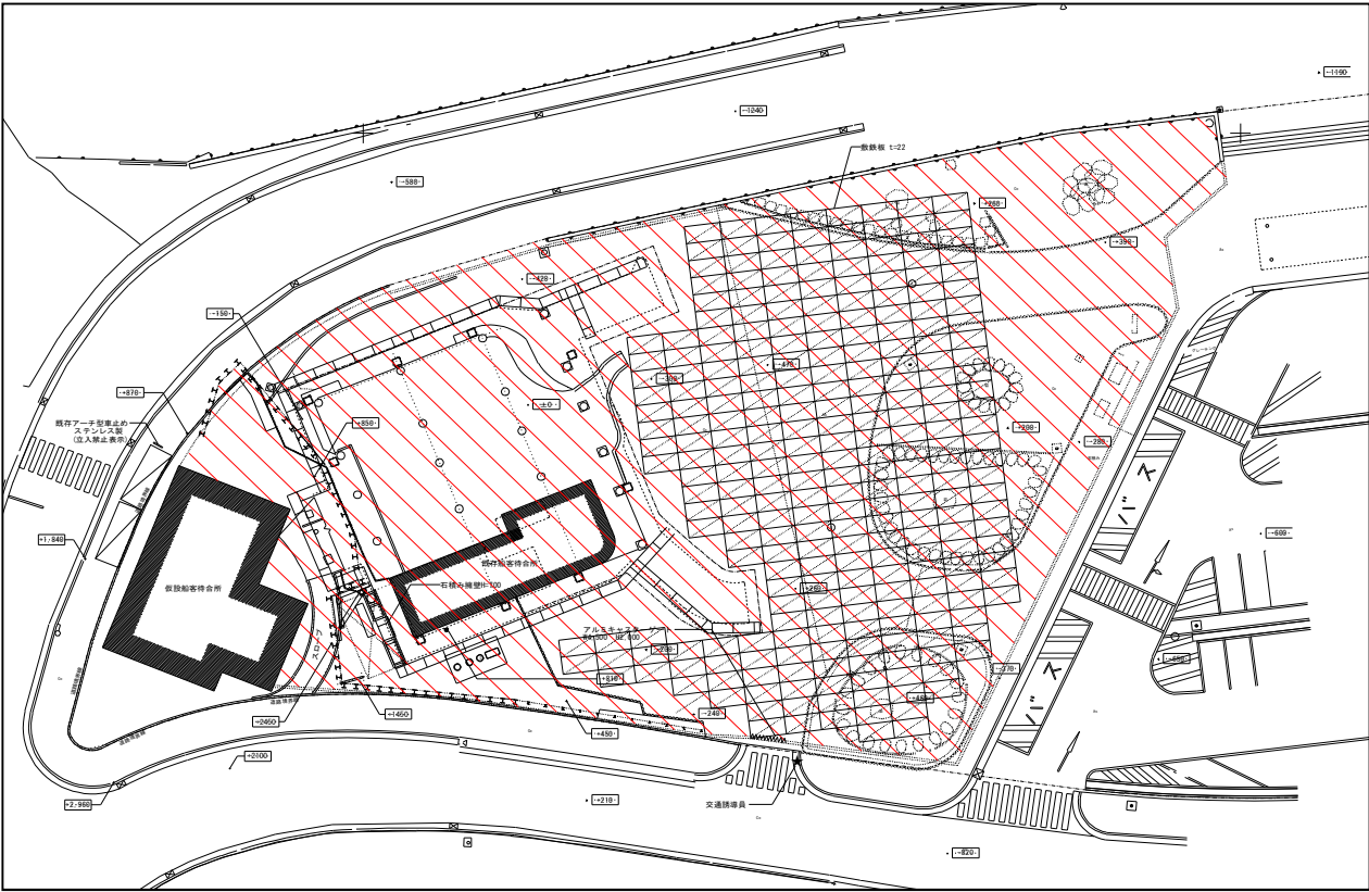
平面図
