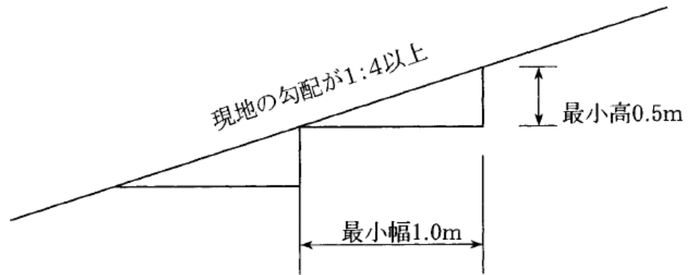
図3.2-1 盛土基礎地盤の段切
