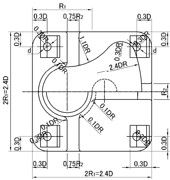
設計けん引力が 50,100,150,250kN の場合
