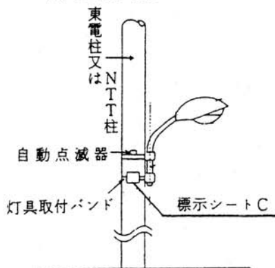
b 街灯Ⅲ型共架ネームプレート
