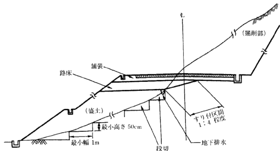
図3.2-2 盛土基礎地盤の段切
