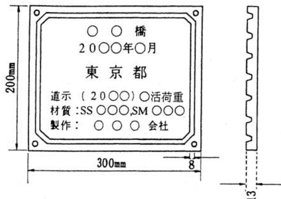
(1) 鋼けた用ネームプレート
