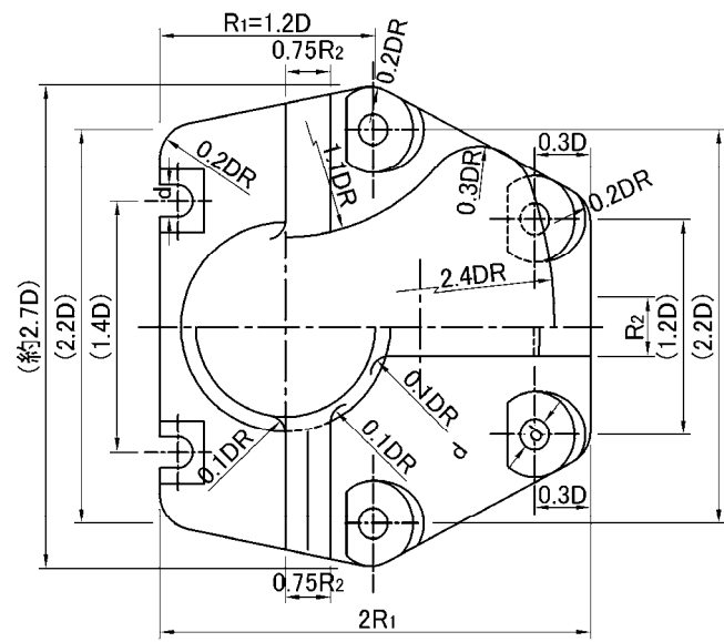
設計けん引力が 350,500,700,1000kN の場合
