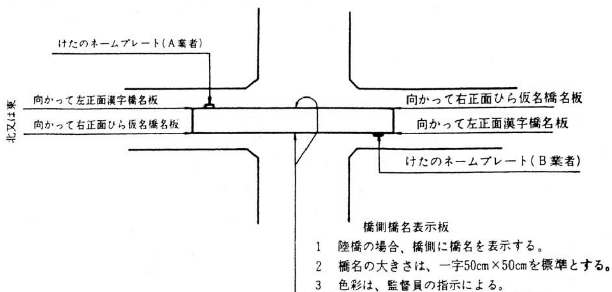
第 2 図 (陸 橋)
